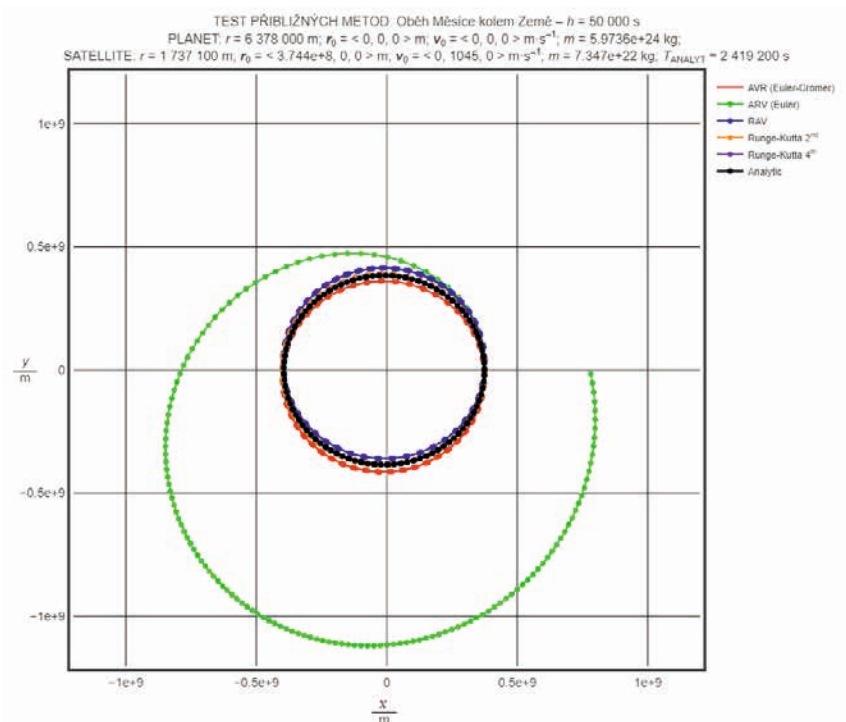
Obr. 5-7 Test přibližných metod: oběh Měsíce kolem Země; h = 50\,000 s
