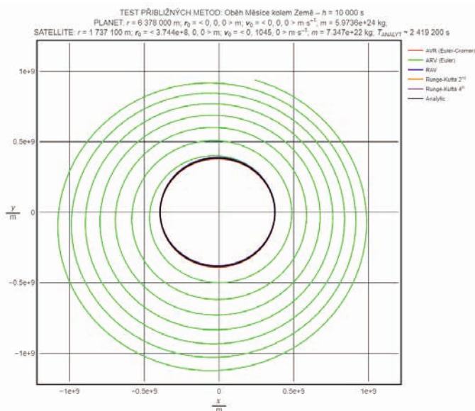
Obr. 5-8 Test přibližných metod: oběh Měsíce kolem Země; h = 10\,000 s
